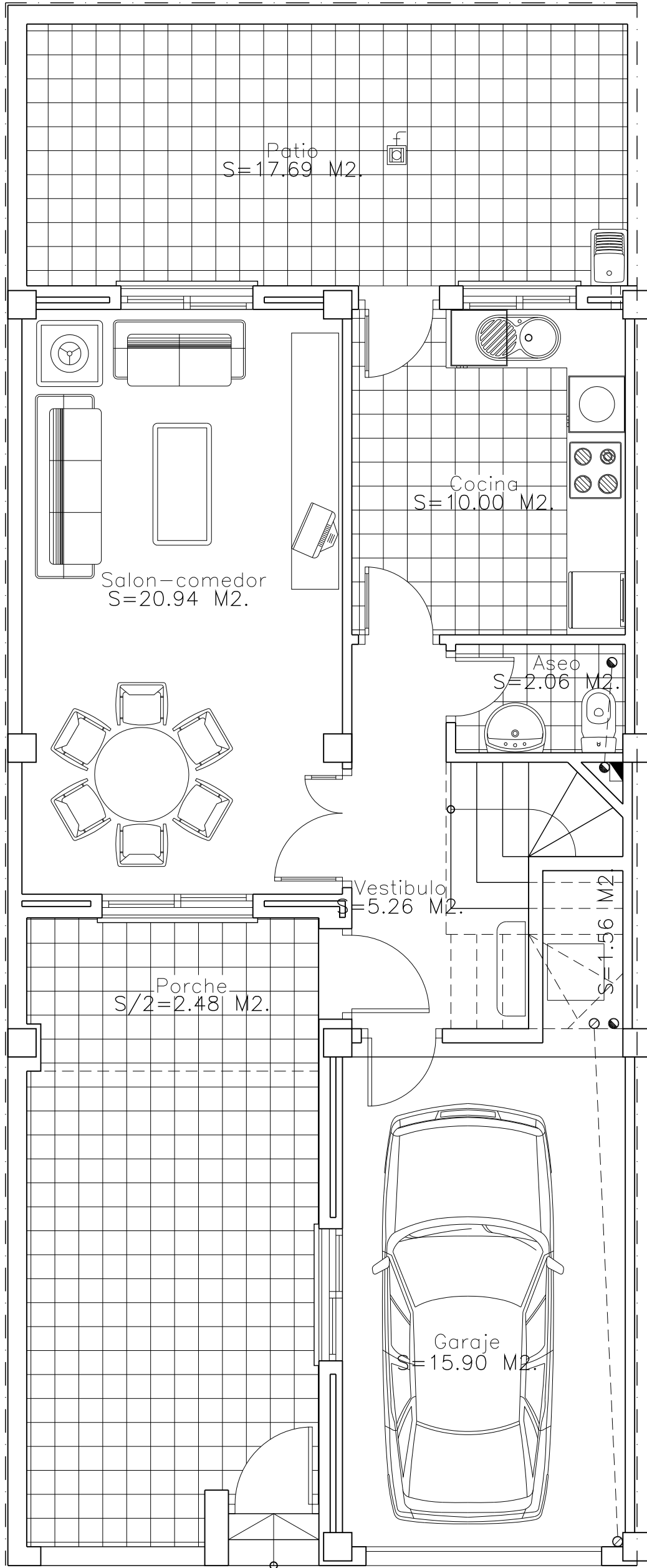
PLANTA BAJA
