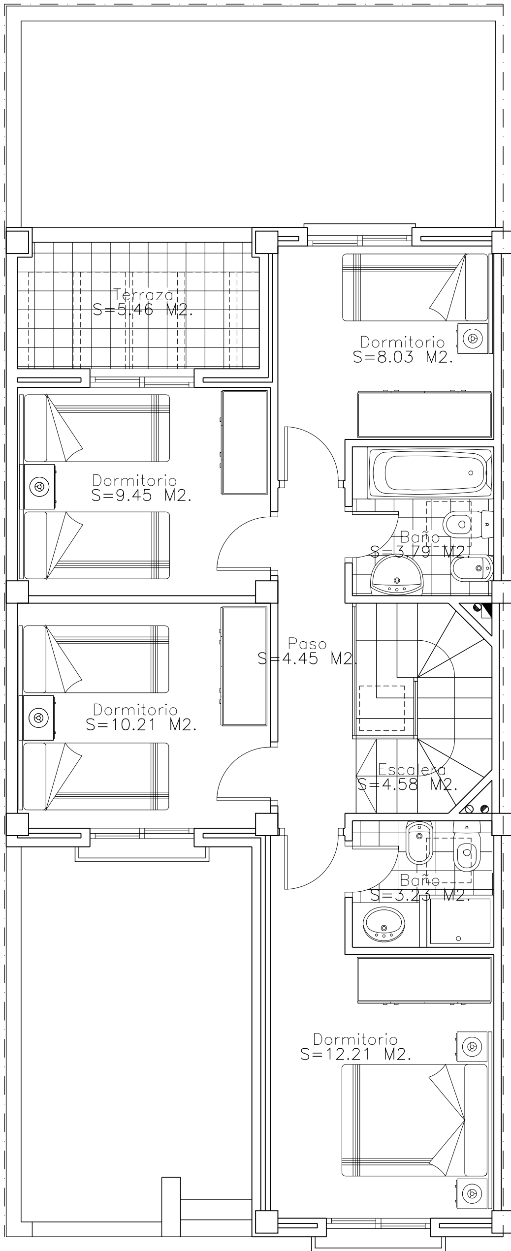
PLANTA ALTA
