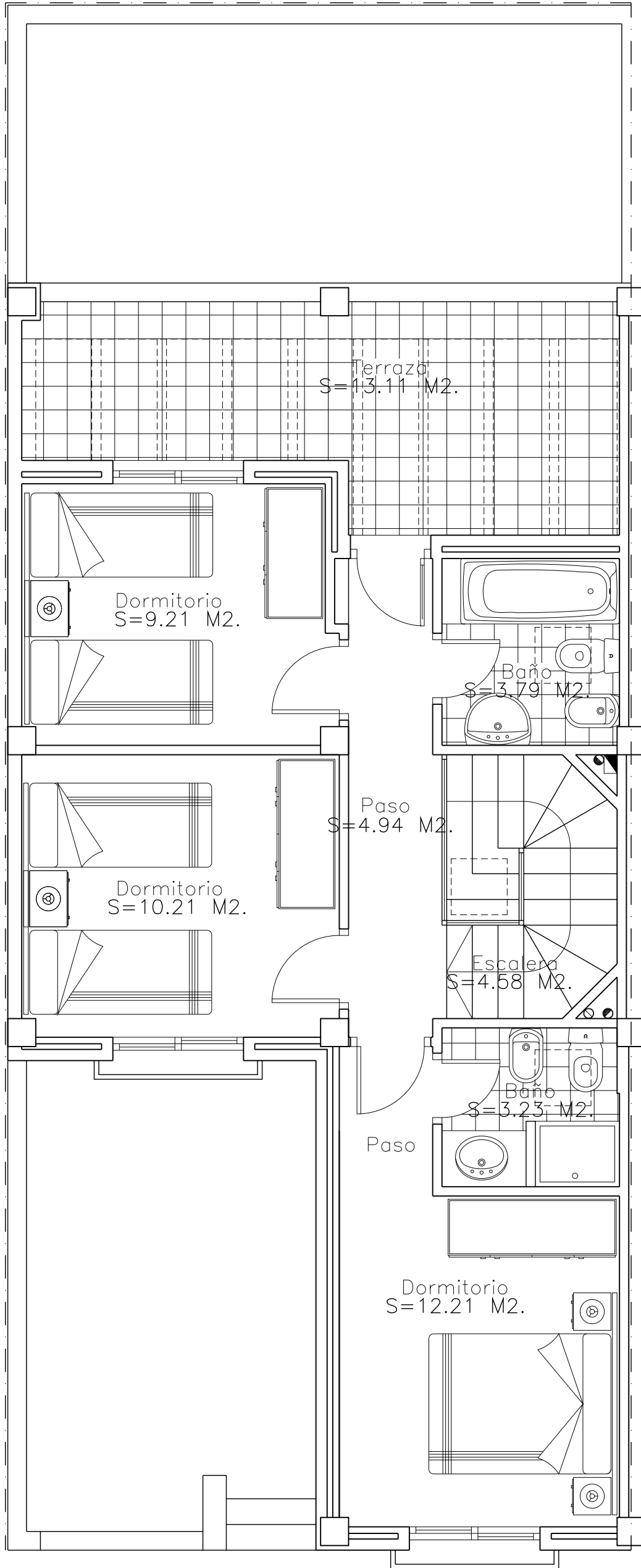
PLANTA ALTA
