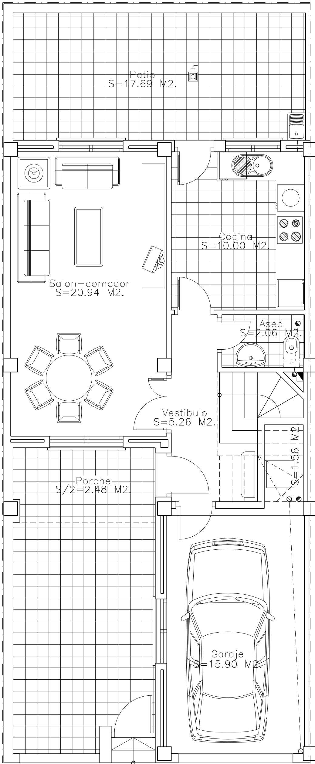
PLANTA BAJA
