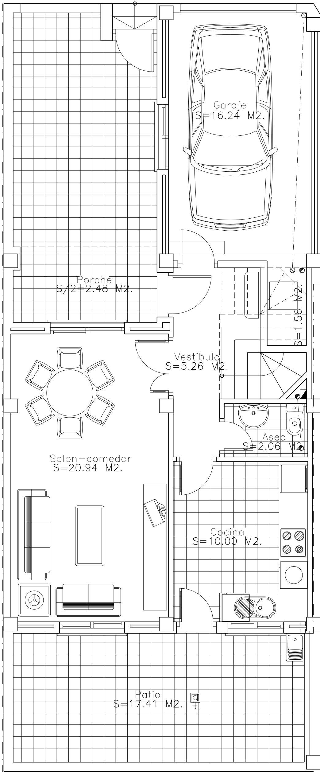
PLANTA BAJA
